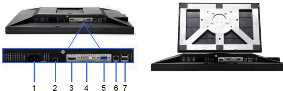
底部図
